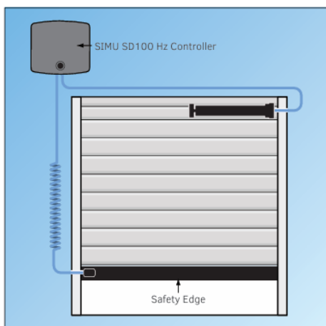
SIMU Safety Edge System
